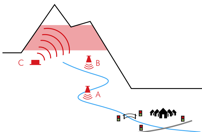
Figure 2 : Système d'alarme pour laves torrentielles (A, B) avec radar de niveau, caméra de surveillance et alarme. Radar interférométrique et caméra de surveillance (C).
