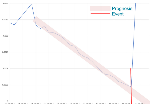
Abbildung 3: Inverse Geschwindigkeitsanalyse mit den Daten der DEFOX™ PRO Kamera. Die Trendkurve weist auf den späteren Abbruchzeitpunkt hin.
