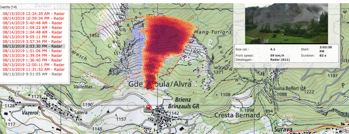
Titelbild: Rutschgebiet.
